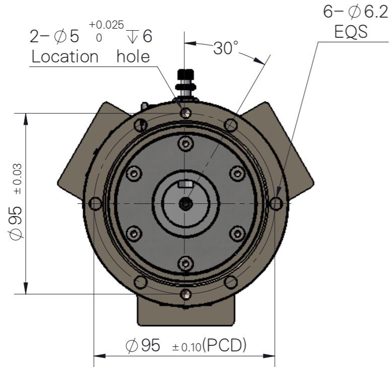
产品名称: 无限连续旋转接头-D95 型号: FY-CRJ-95-F
