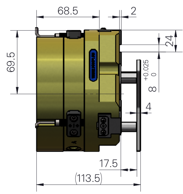
带推料装置图
